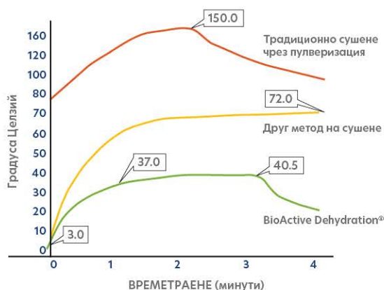
Графиката изобразява точната и приблизителна температура на продукта в продължение на 4 минути при най-често срещаните процеси на сушене на водораслите. Резултатите могат да варират в зависимост от различните производствени практики.
